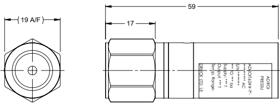
CONSTRUZIONE PER BASSE PRESSIONI (CAMPI DI MISURA <10 BAR)
