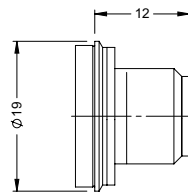
CONNETTORE M12X1 4-PIN PER ALTA TEMPERATURE (TD)
