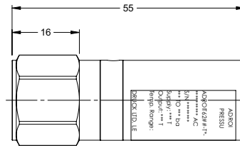
CONSTRUZIONE PER CAMPI MEDI (CAMPI DI PRESSIONE > 10 BAR A > 350 BAR)
