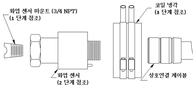
화염 센서와 수냉 자켓 설치 안내
