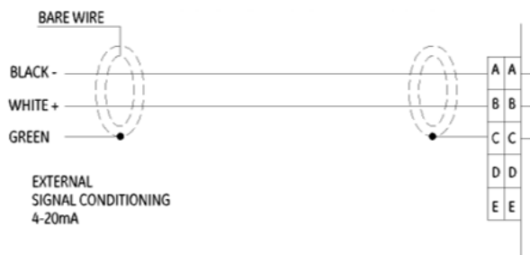
МОНТАЖНАЯ СХЕМА SiC ДАТЧИКА ПЛАМЕНИ FLAME TRACKER™
